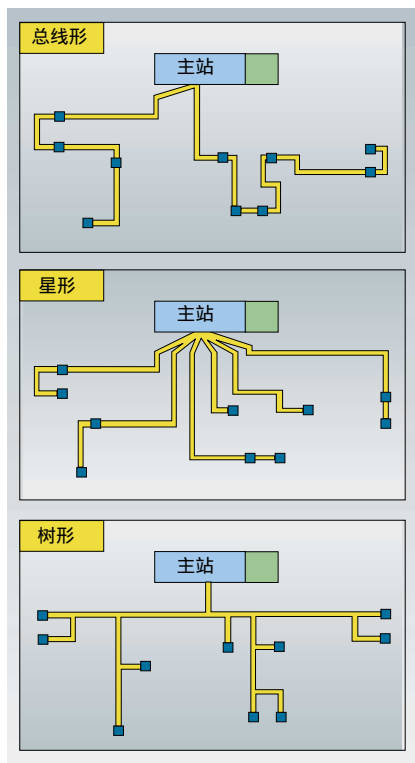
AS interface 网络可以配置成总线形，星形或树形结构。
