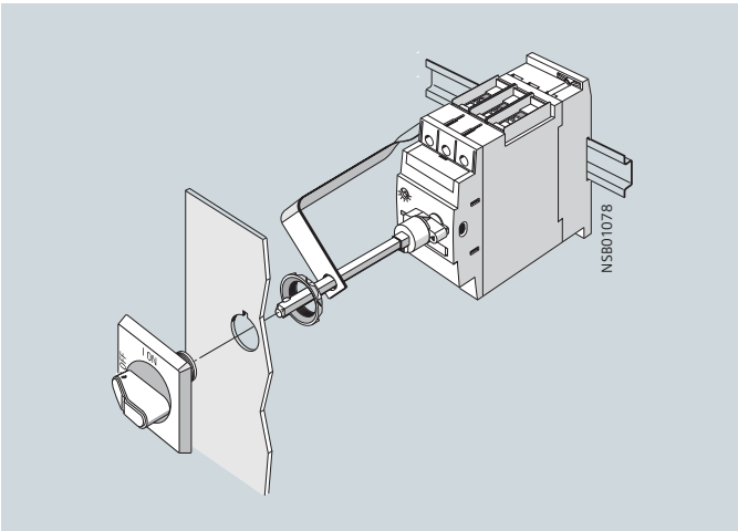
图：3RV69 26-0K 门耦合旋转操作机构
