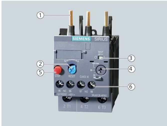
图：3RU61 26 热过载继电器
