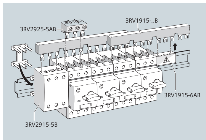
图：三相母线系统（S00/S0 规格为例）
