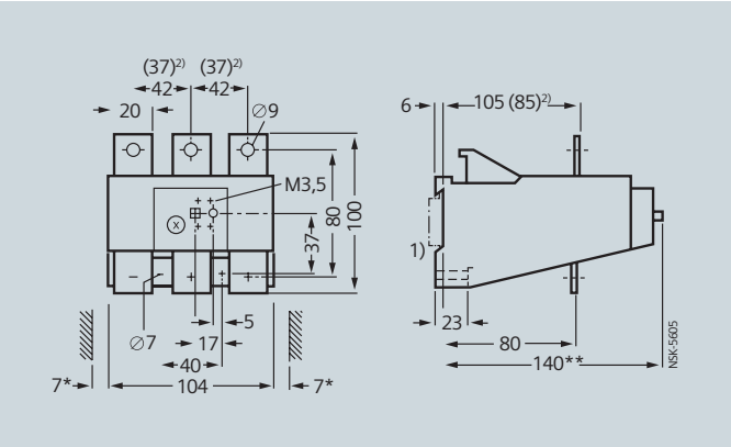
3UA62 40-.. 独立安装
