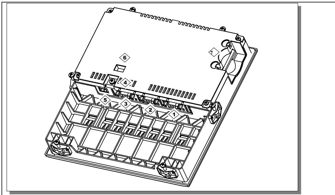
图9-3 连接元素的布置
