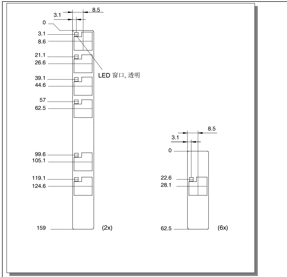
图10-4 标签条尺寸
