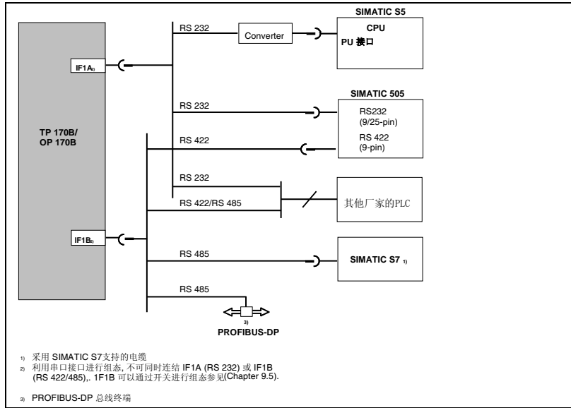
图9-7 PLC 的连接配置
